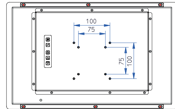
Rückansicht
