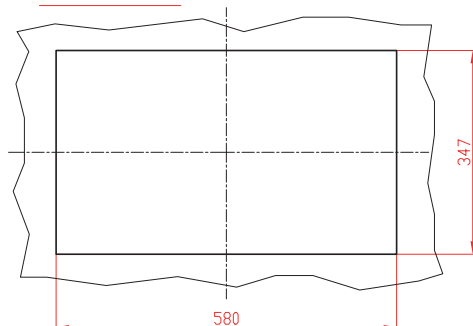
FRONTANSICHT
