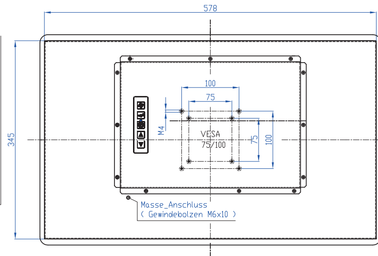
RÜCKANSICHT
