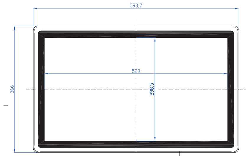
FRONTANSICHT
