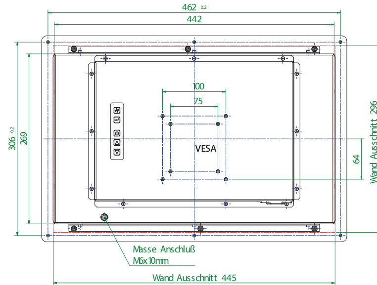
Rückansicht
