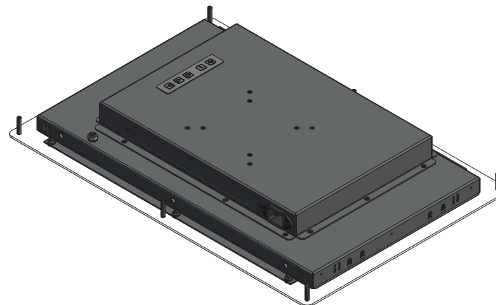
Rückansicht
