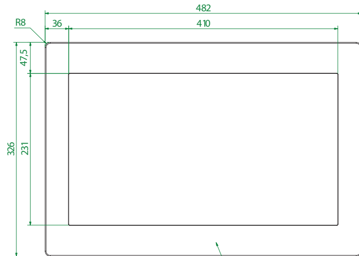
Frontansicht
